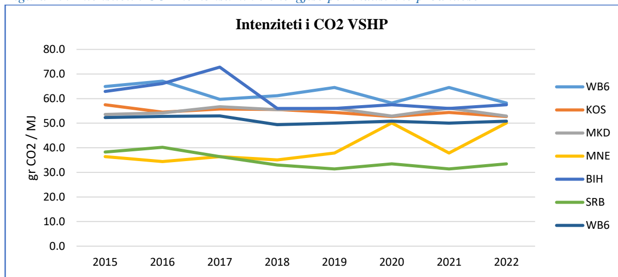
Figura 13: Intesiteti i CO2 në konsumin e energjisë për industrinë prodhuese
