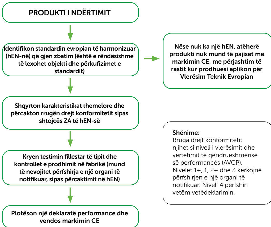
Figura 2: Diagrami i vlerësimit të konformitetit me pesë hapa për produktet e ndërtimit
